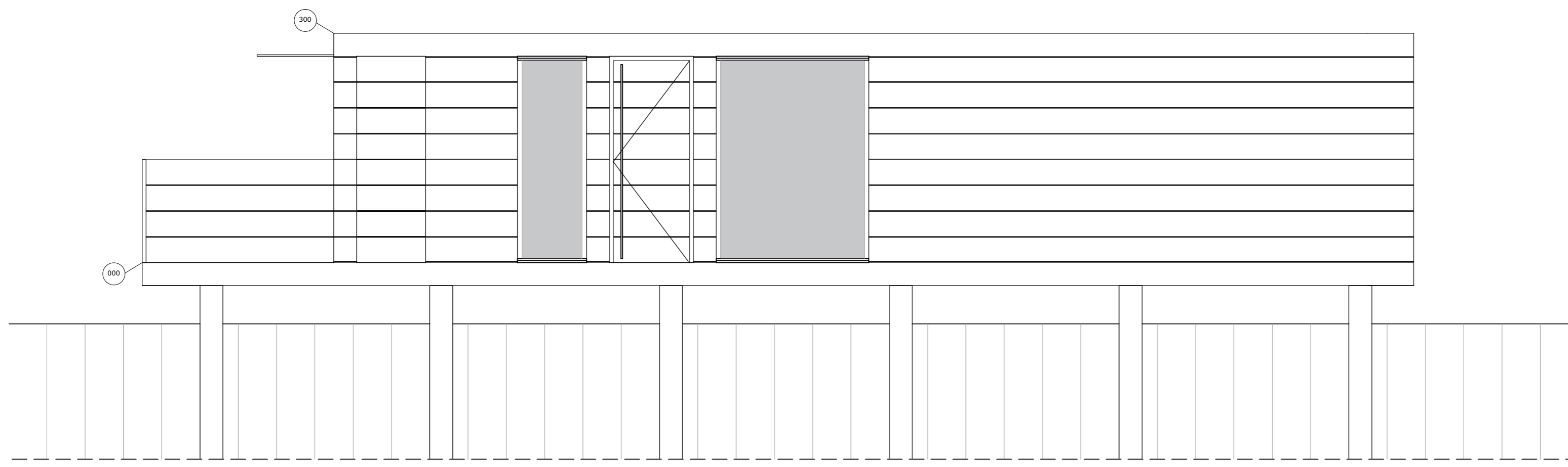
VOORGEVEL 1:50
